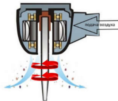
НАКОНЕЧНИК НТКС-300-1 СЗМ С СИСТЕМОЙ CLEAN HEAD
