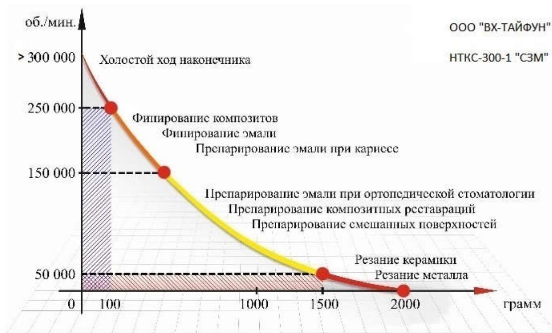
График эффективной работы турбинного наконечника НТКсд-300.
